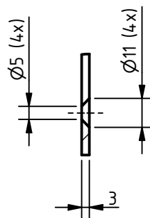
B ( 1 : 2 )
