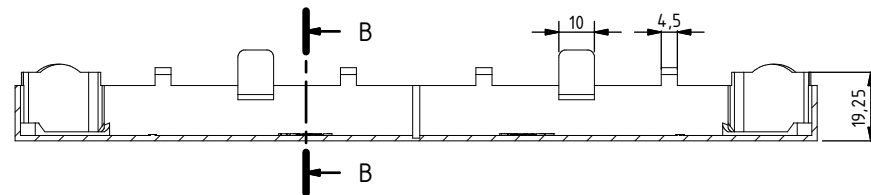
A-A ( 1 : 1.5 )
