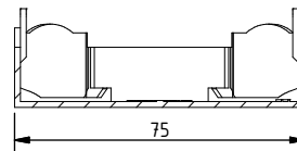
B-B ( 1 : 1.5 )
